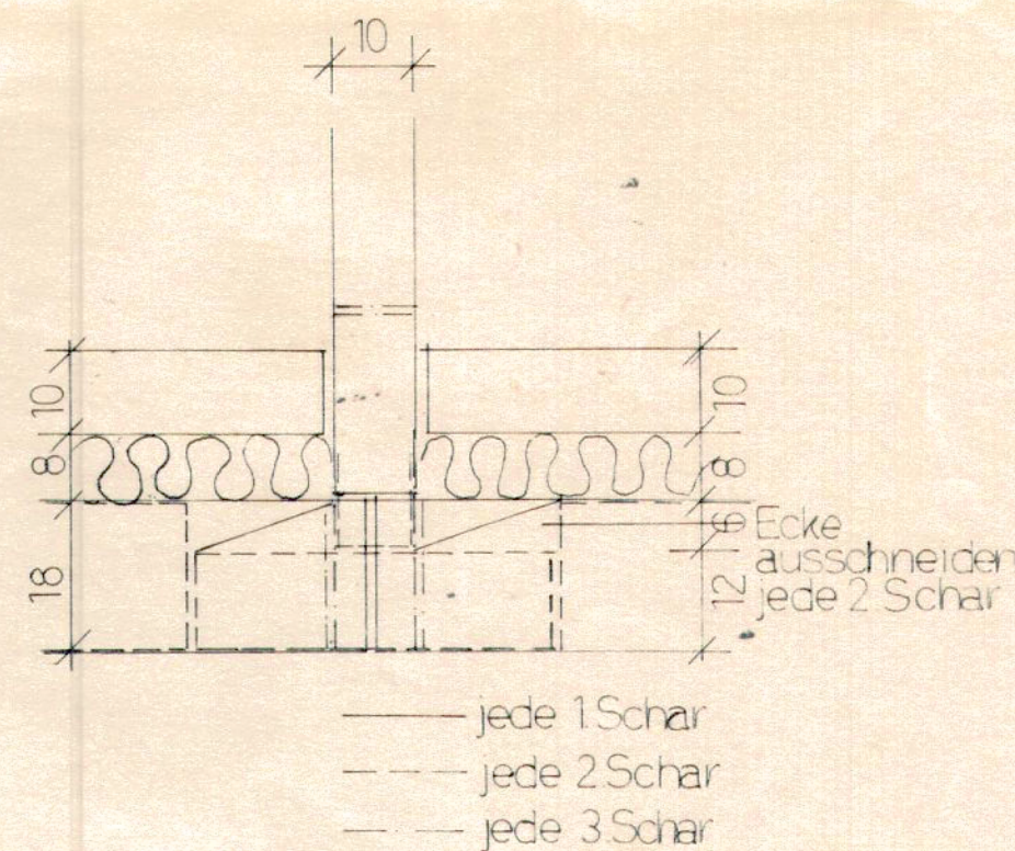
DETAIL A Trennwandanschluss 1:10
