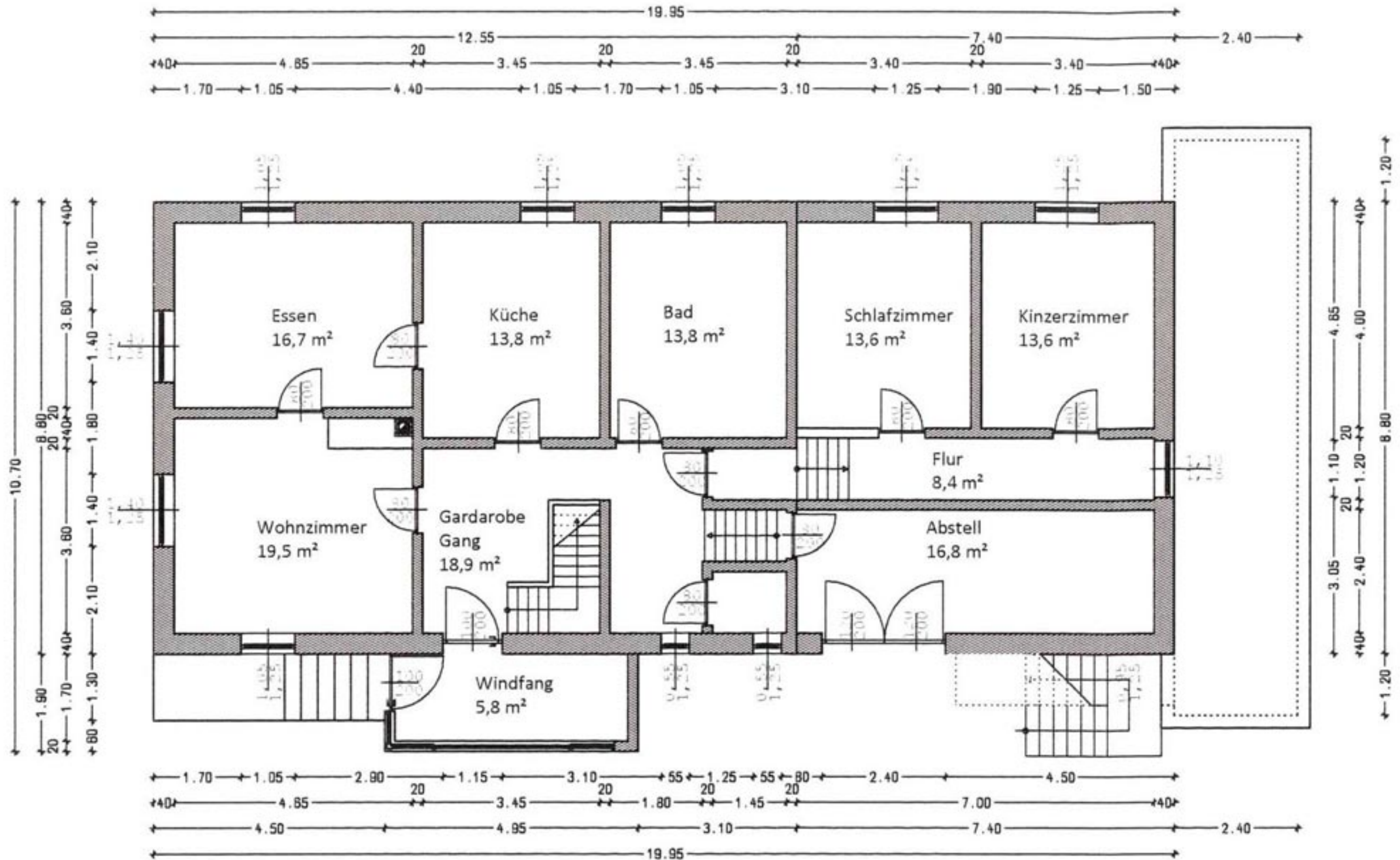
Erdgeschoss 1:100
